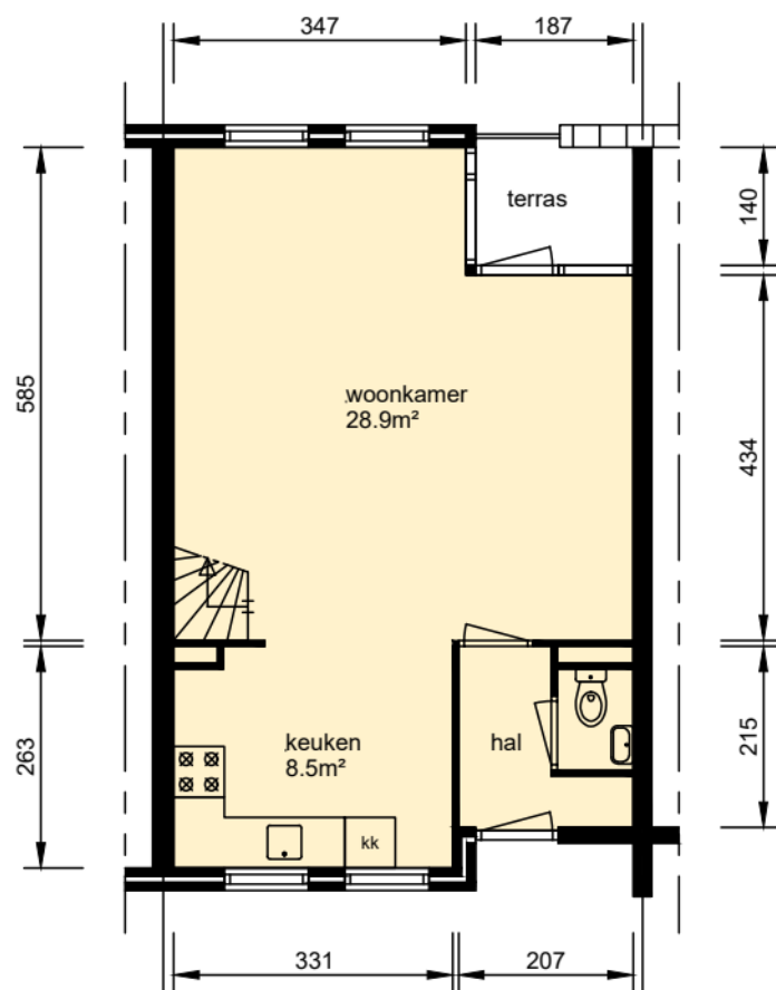
1e verdieping
