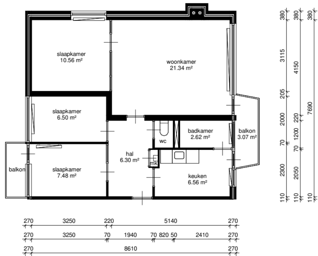
eerste verdieping
