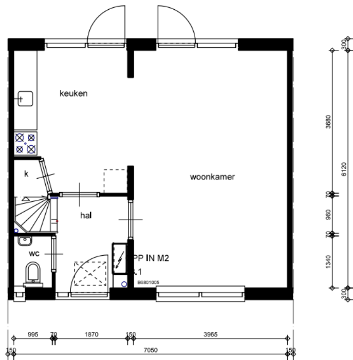
BEGANE GROND
