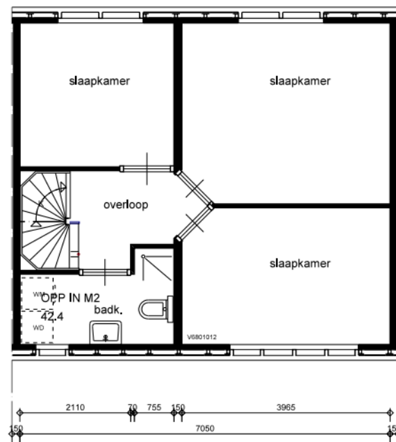
1e VERDIEPING
