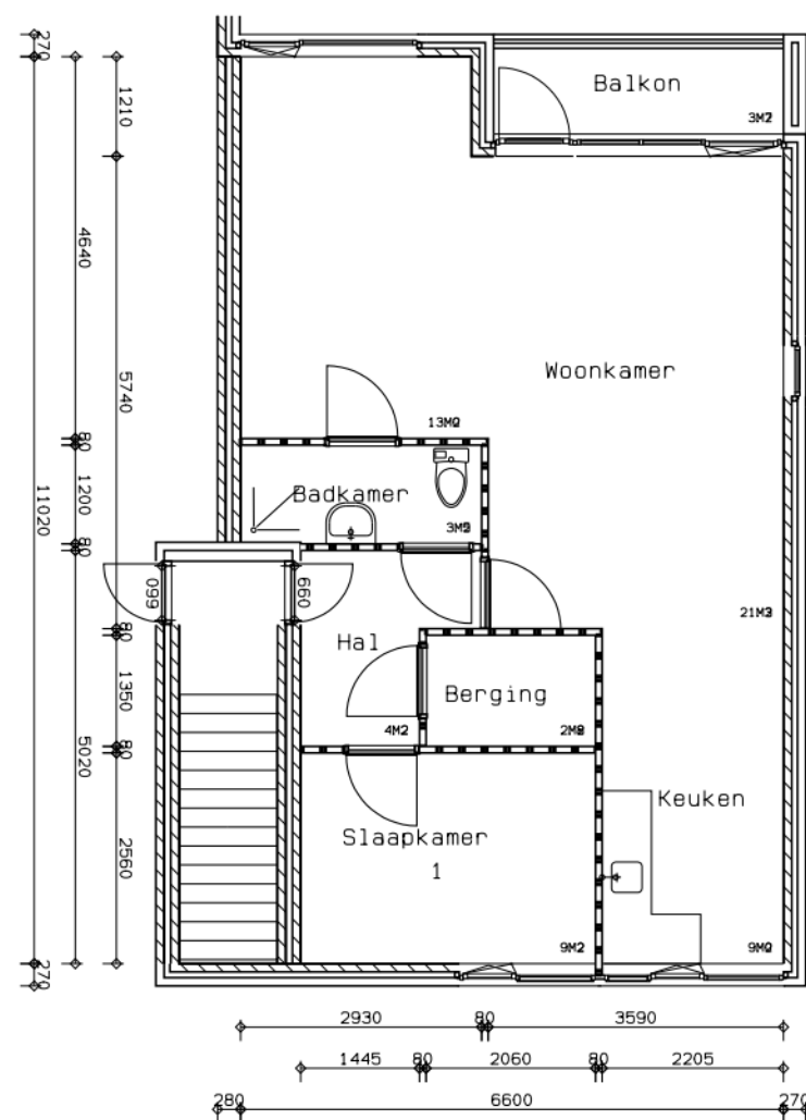
Verdieping
