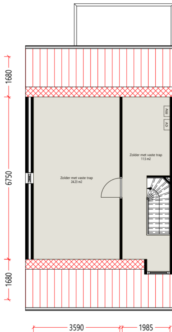
Verdieping_1e
