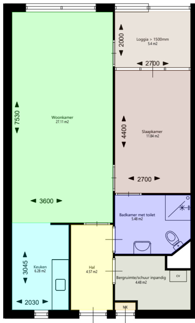
Verdieping_3e
