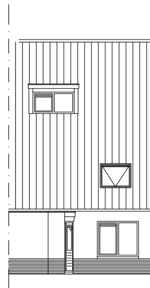
Achtergevel
