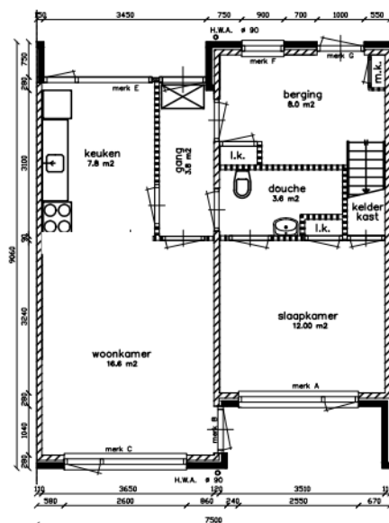
Begane-grond Tussenwoning
