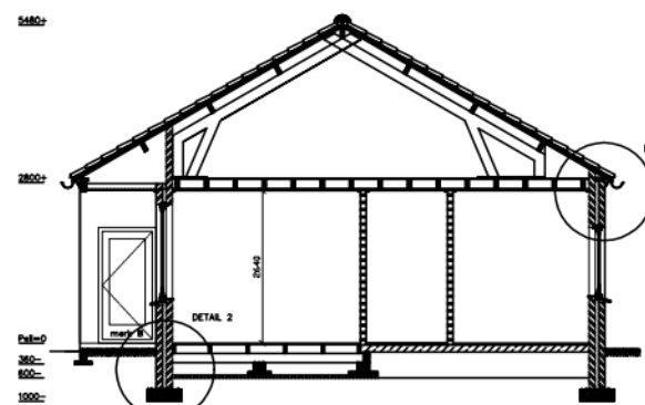
DOORSNEDE schaal 1:50
