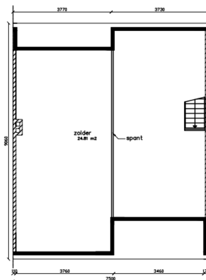
Verdieping Tussenwoning
