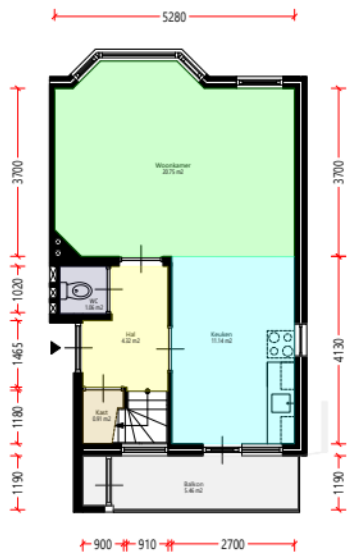
Verdieping_2e
