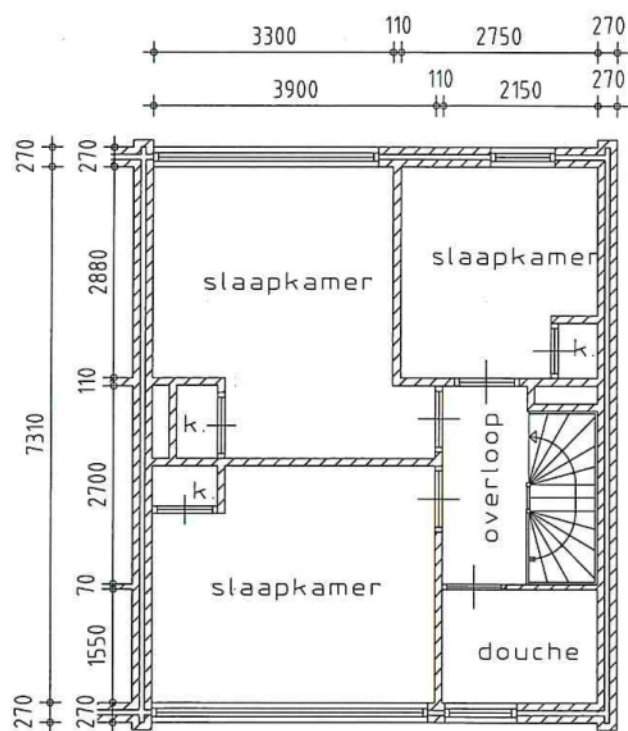
verdieping
