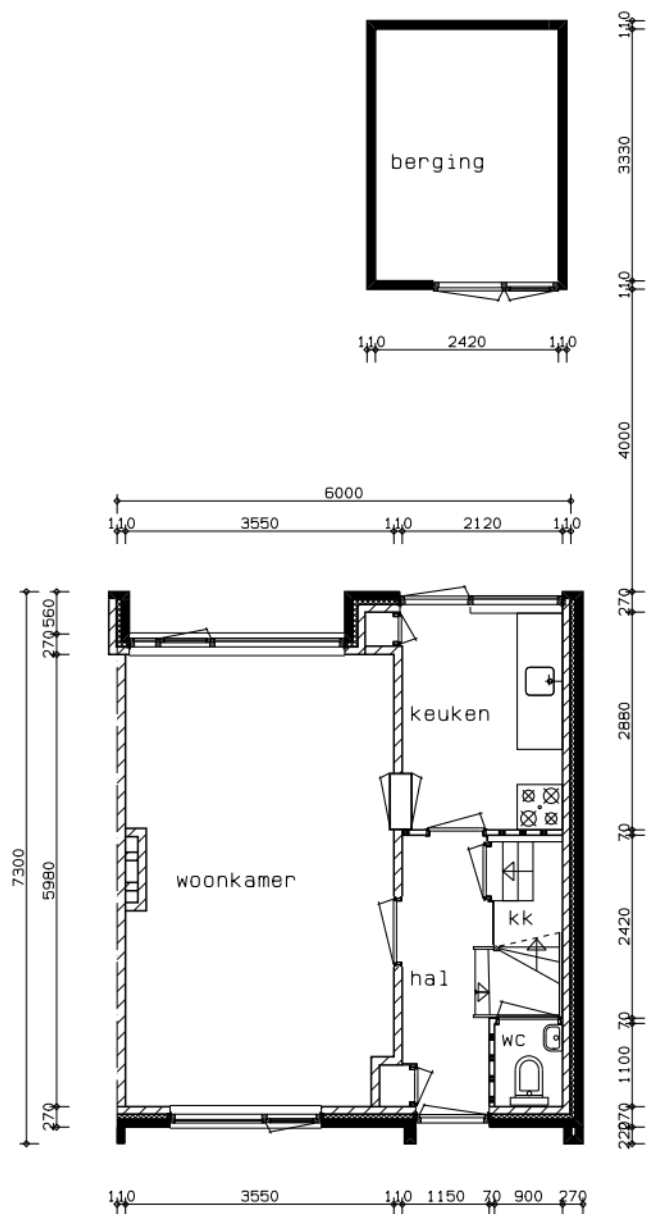
BEGANE GROND
