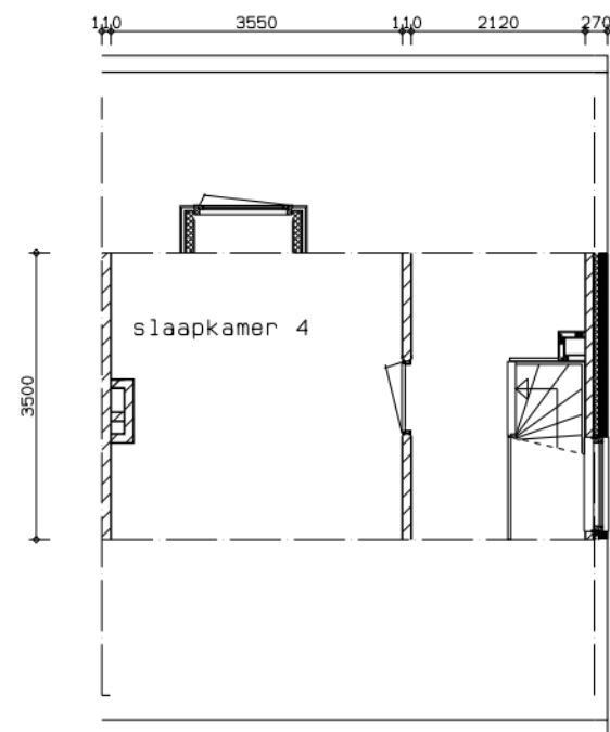
2e VERDIEPING
