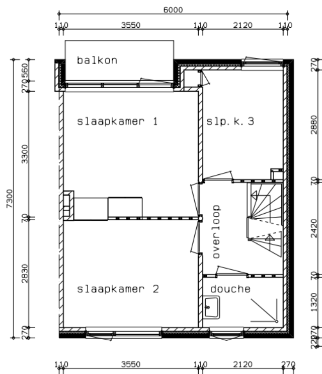
1e VERDIEPING
