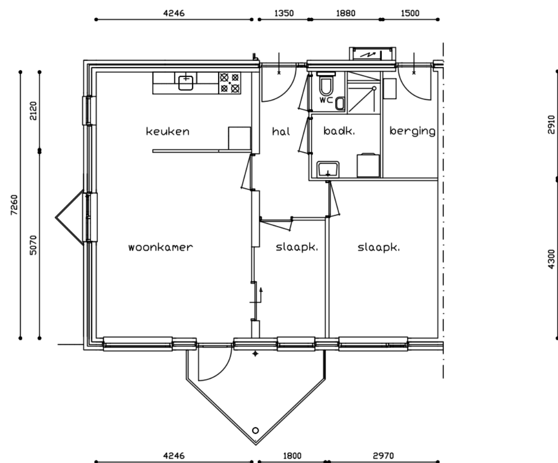
Plattegrond
