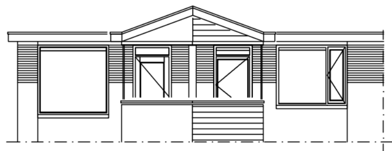
Gevelfragment
