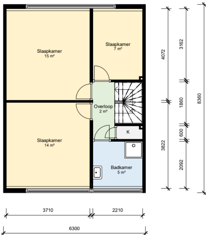
01 Eerste verdieping
