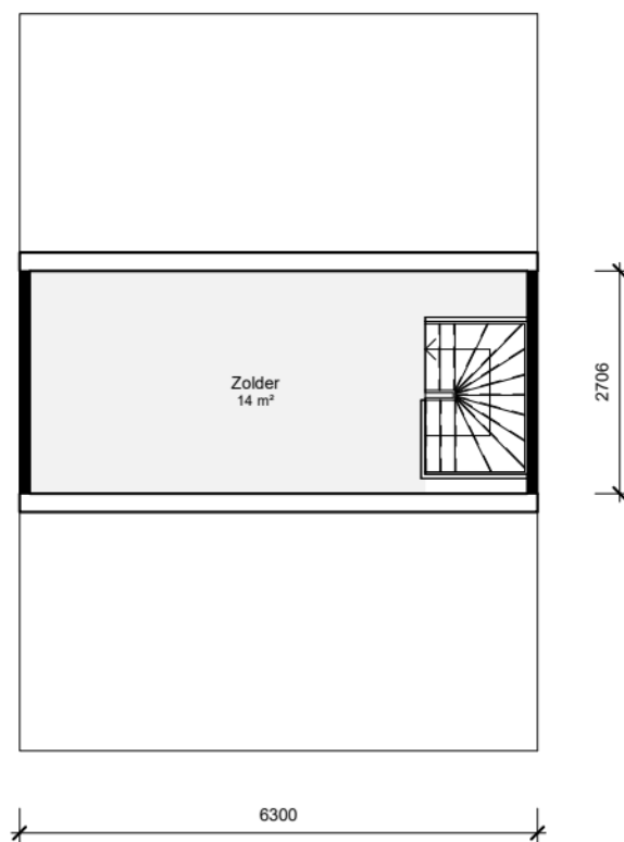
02 Tweede verdieping
