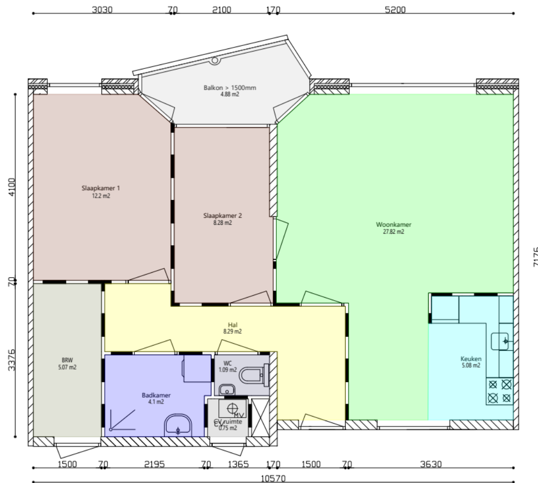
Verdieping_2e
