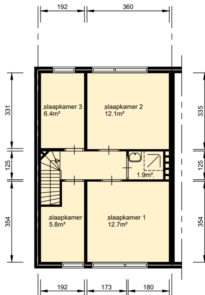
verdieping
