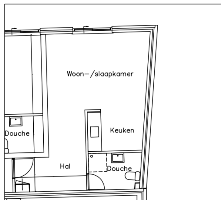
Plattegrond
