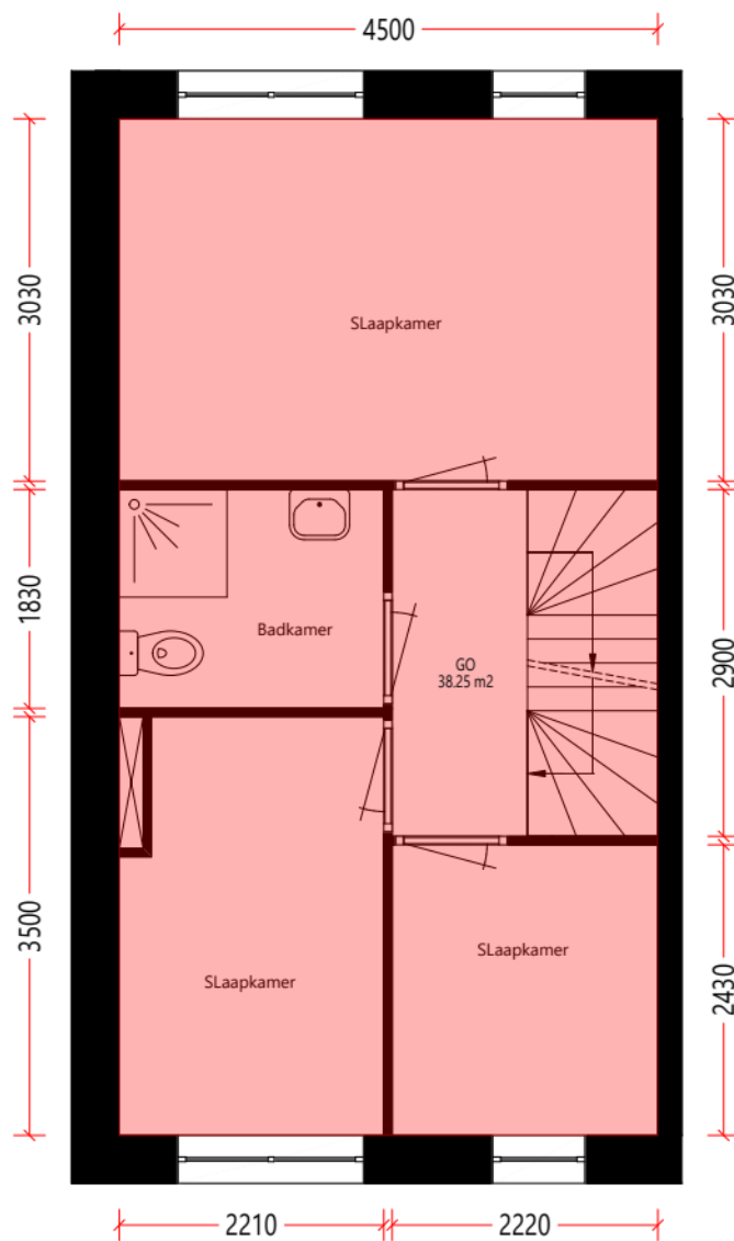
Verdieping_1e
