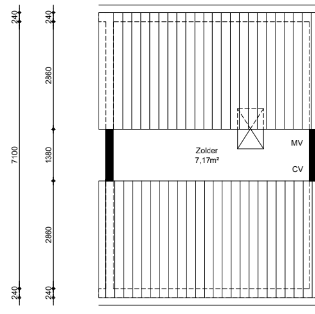
2e verdieping
