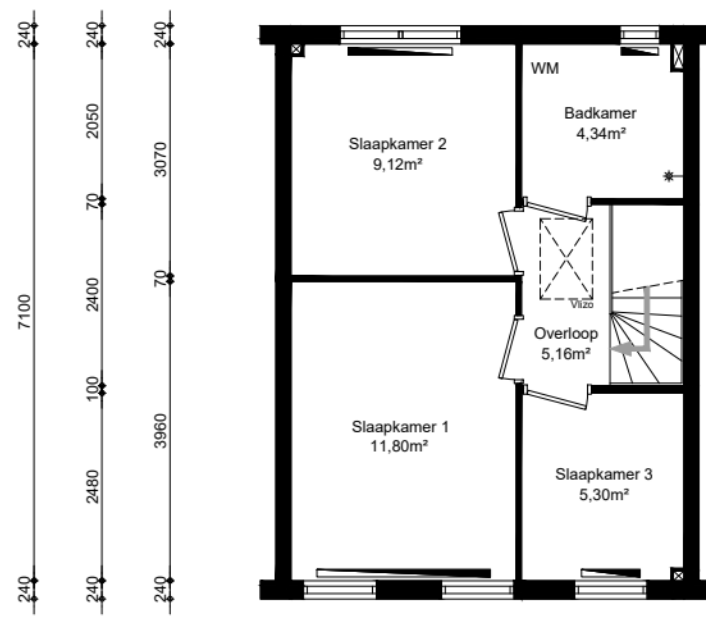
1e verdieping
