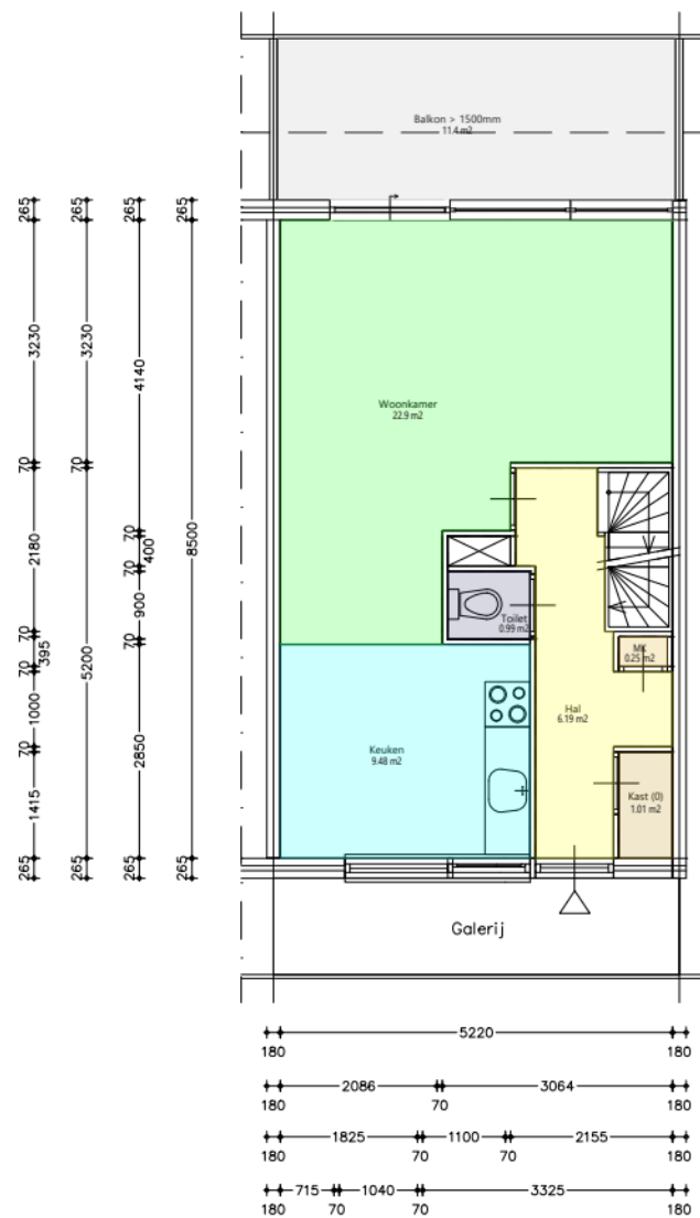
Verdieping_1e
