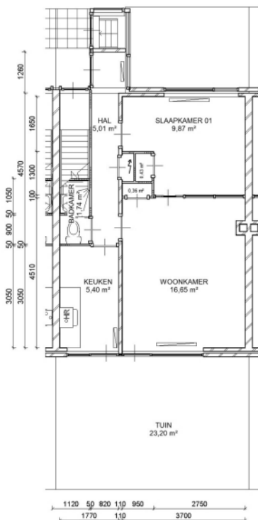
Begane grond
