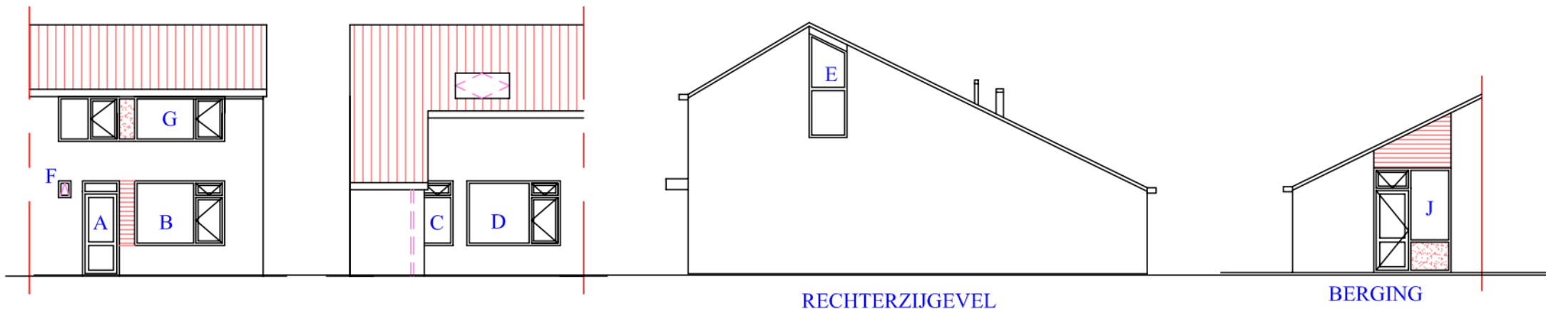
VORGEVEL
