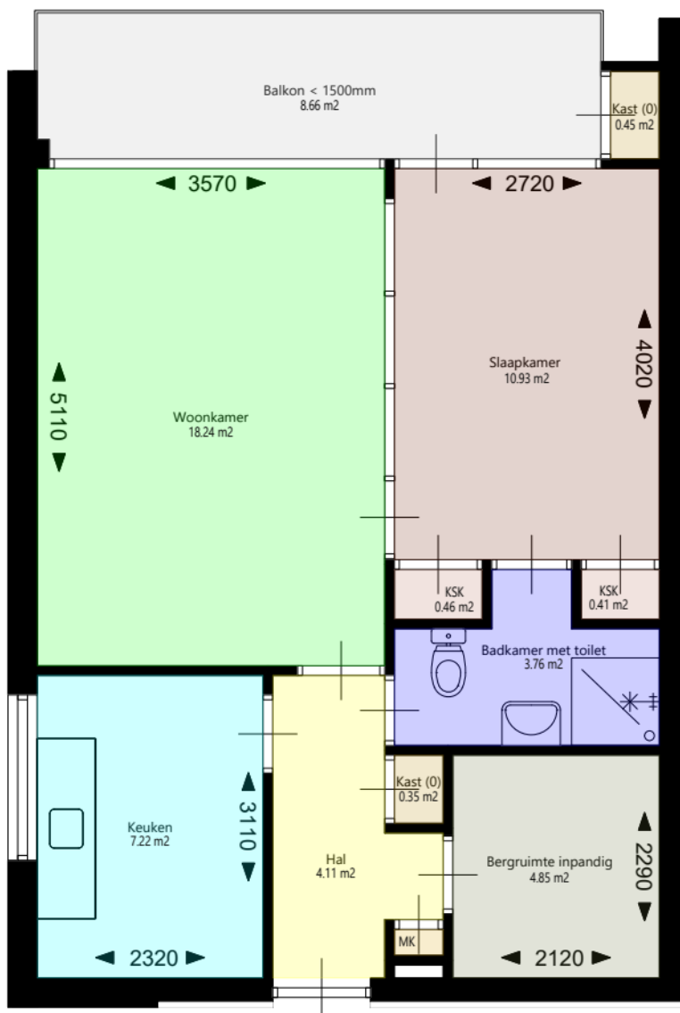
Verdieping_1e
