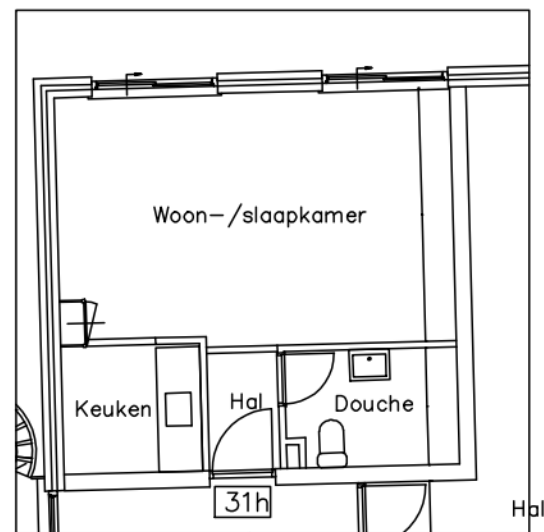
Plattegrond
