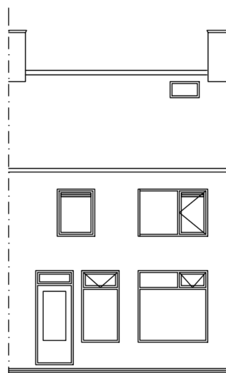
Achtergevel
