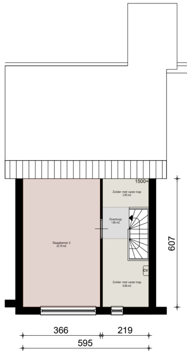
Verdieping_1e
