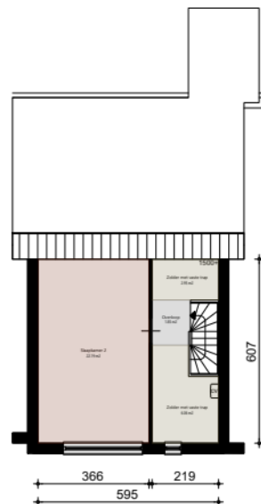
Verdieping_1e
