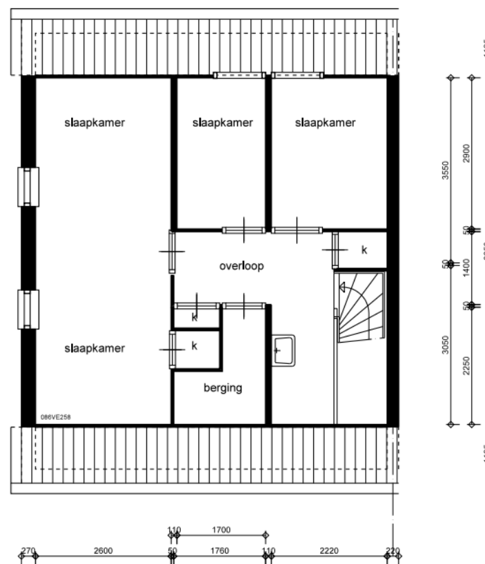
VERDIEPING
