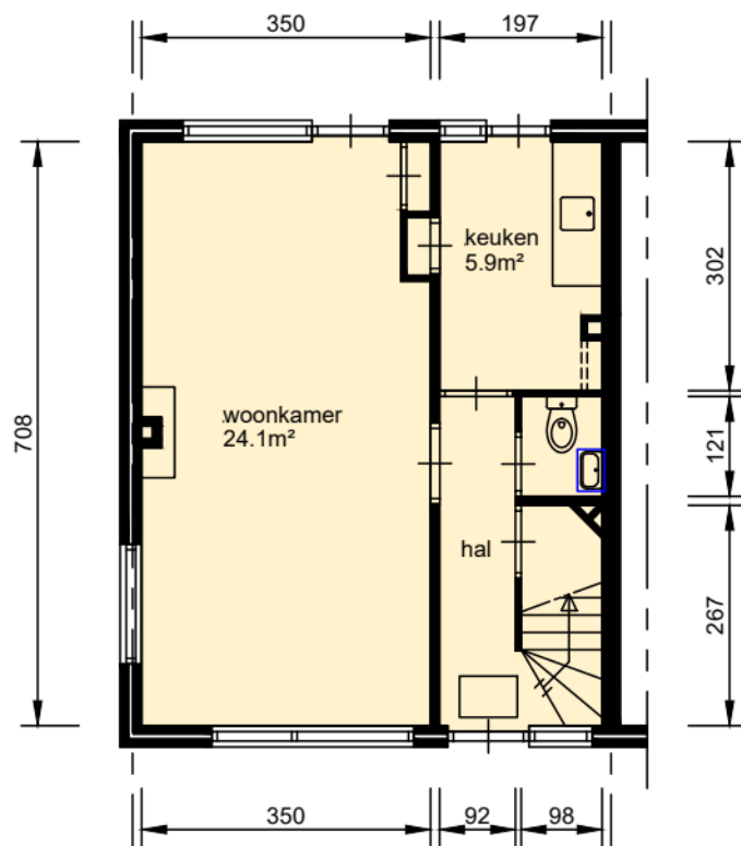
begane grond
