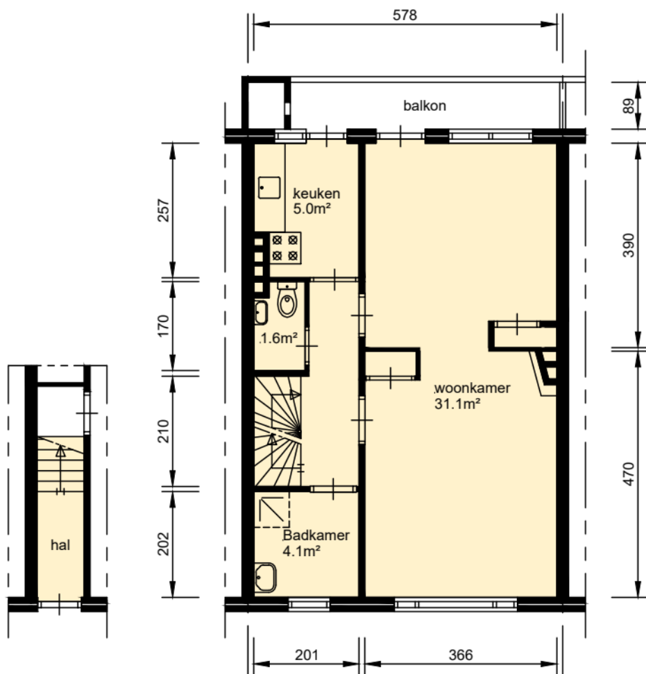
begane grond
