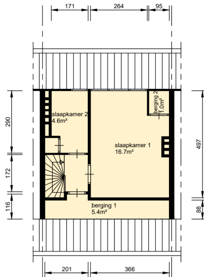
2e verdieping
