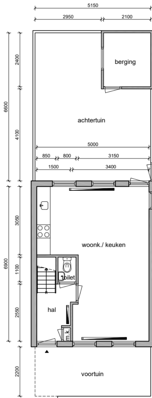
Begane grond
