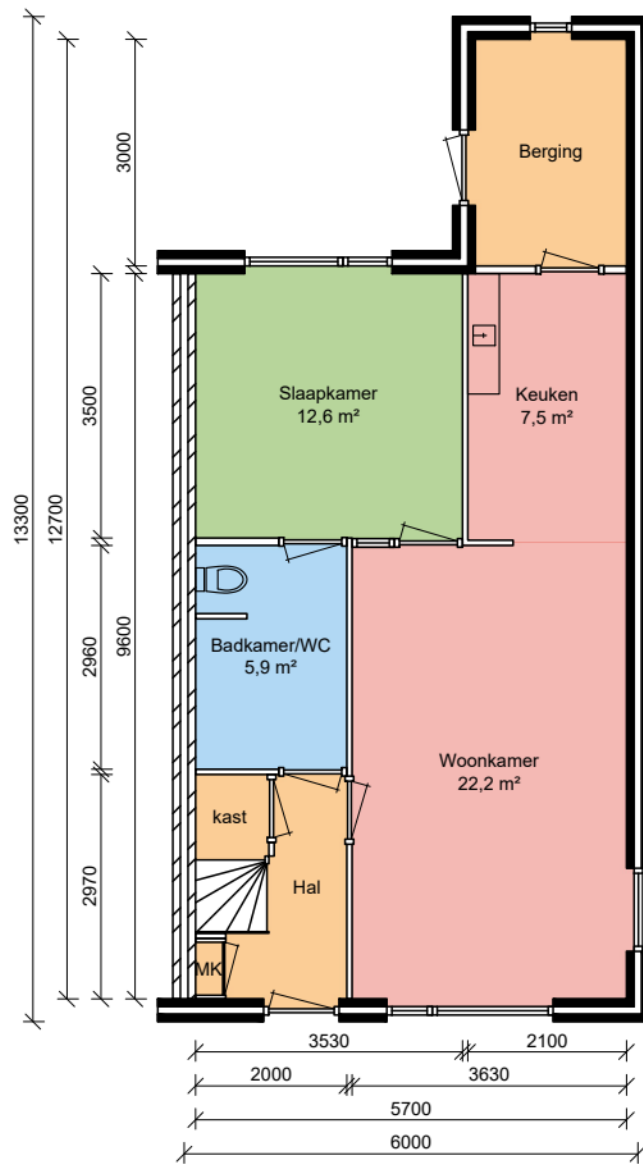
Begane grond
