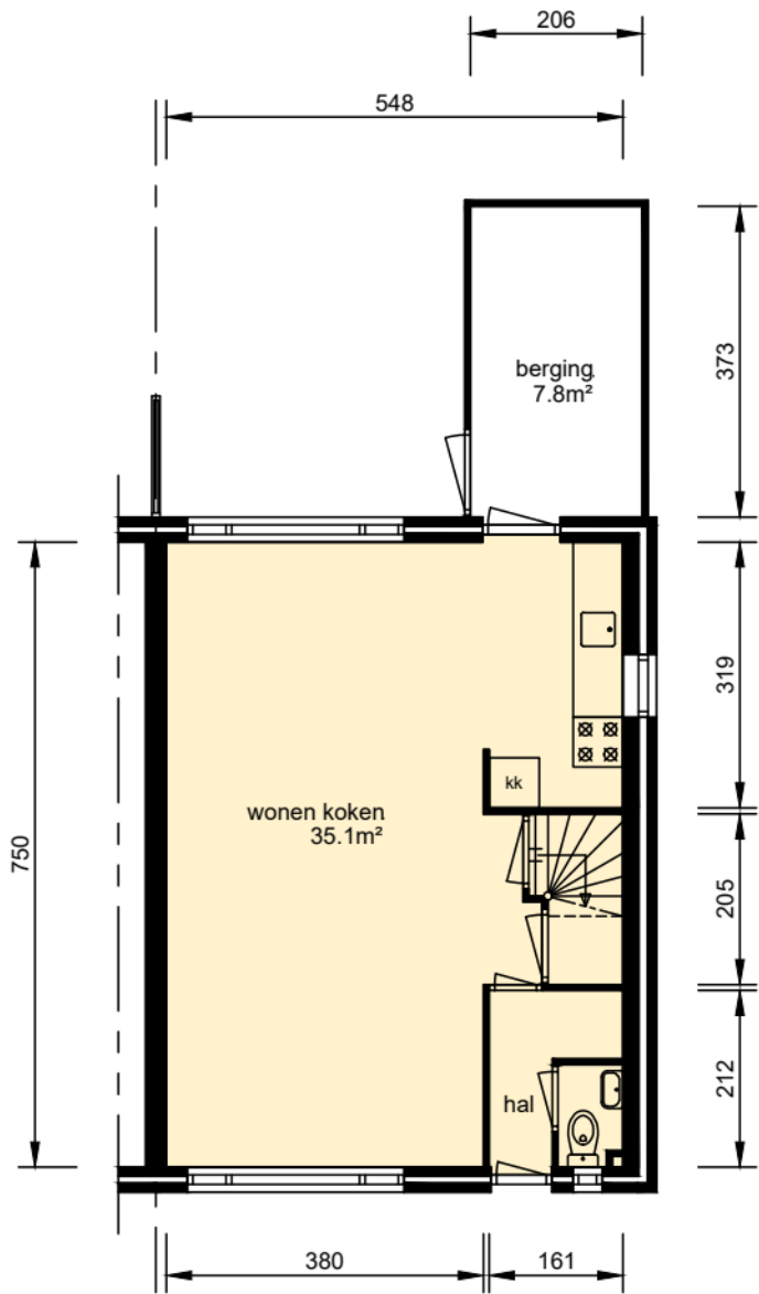
begane grond
