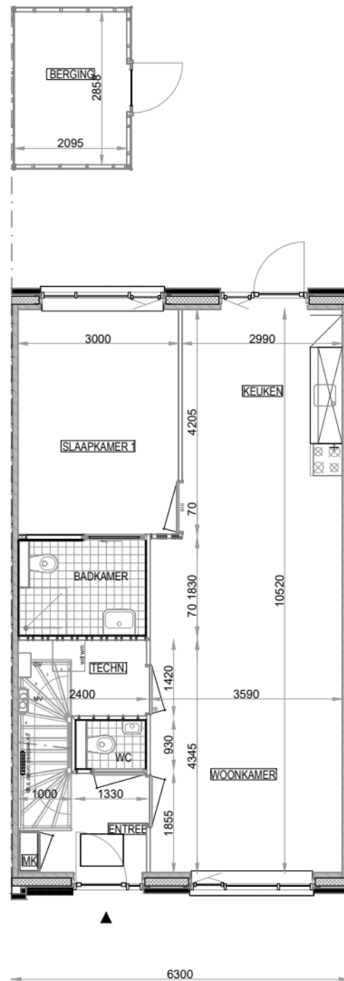
BEGANE GROND
