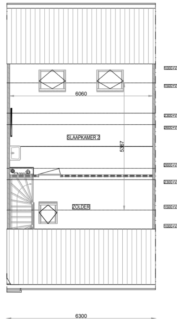
EERSTE VERDIEPING
