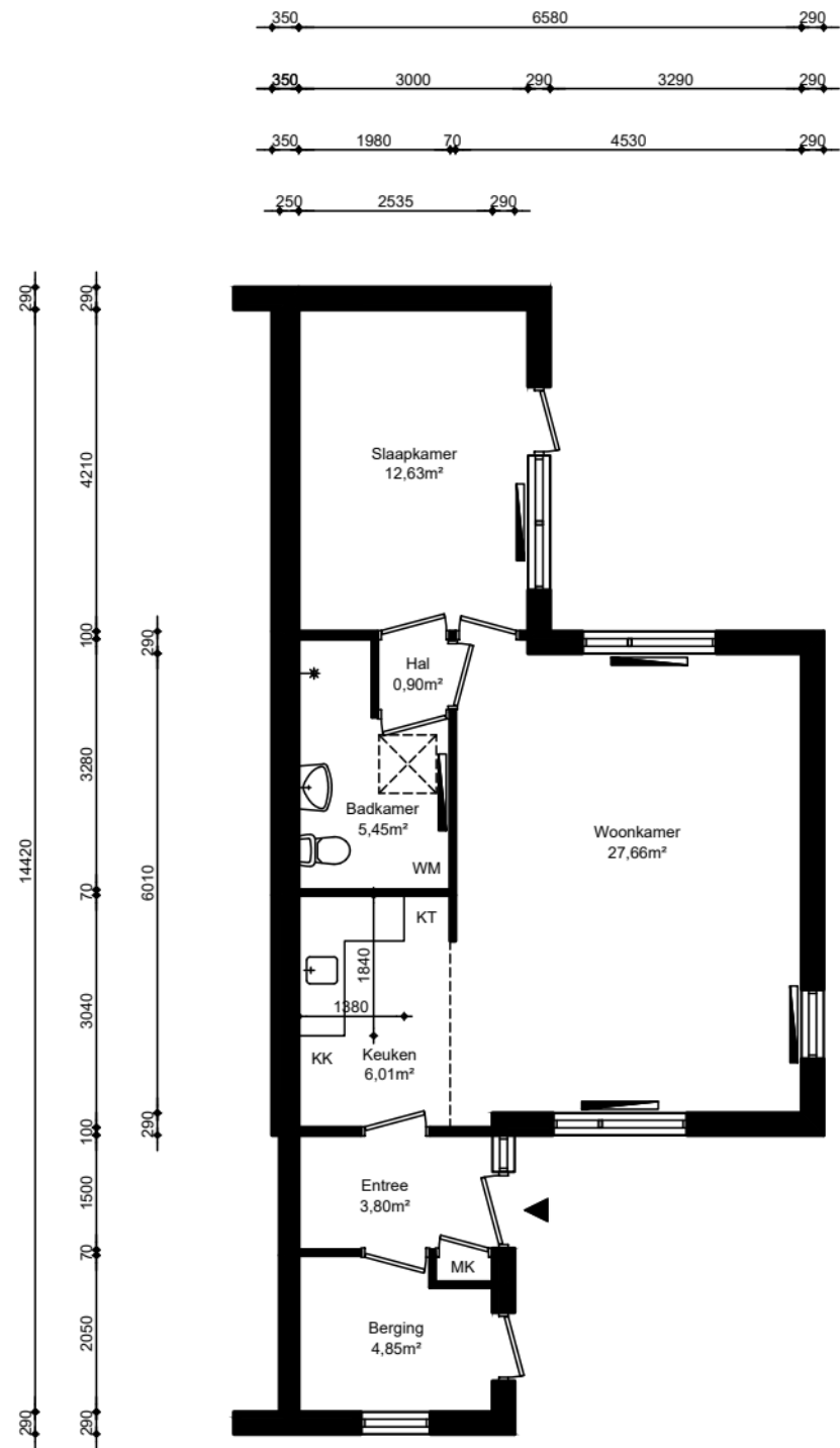
Begane grond
