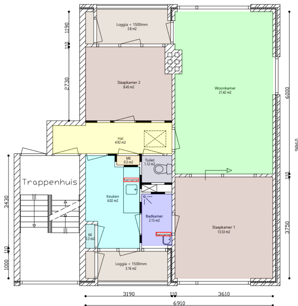
Verdieping_3e
