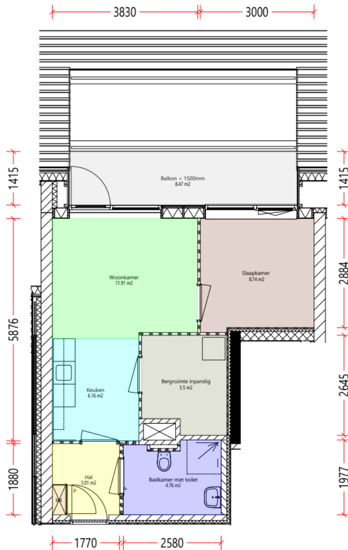
Verdieping_2e
