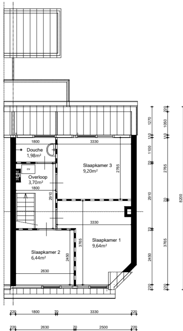
Verdieping
