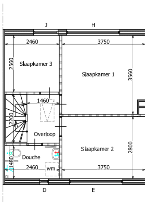
1e verdieping
