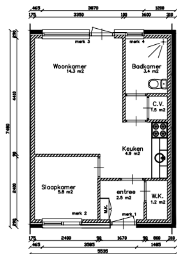
Hoekwoning Begane-grond
