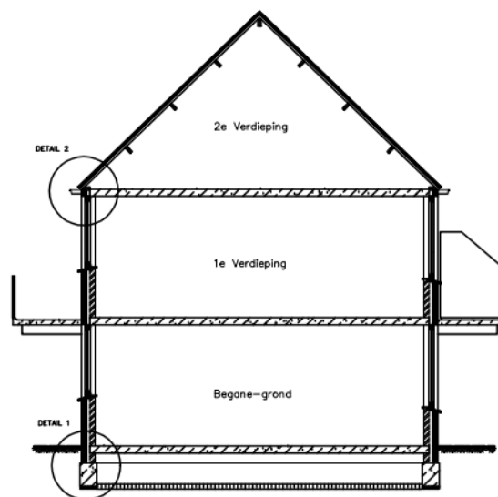
DOORSNEDE A-A
