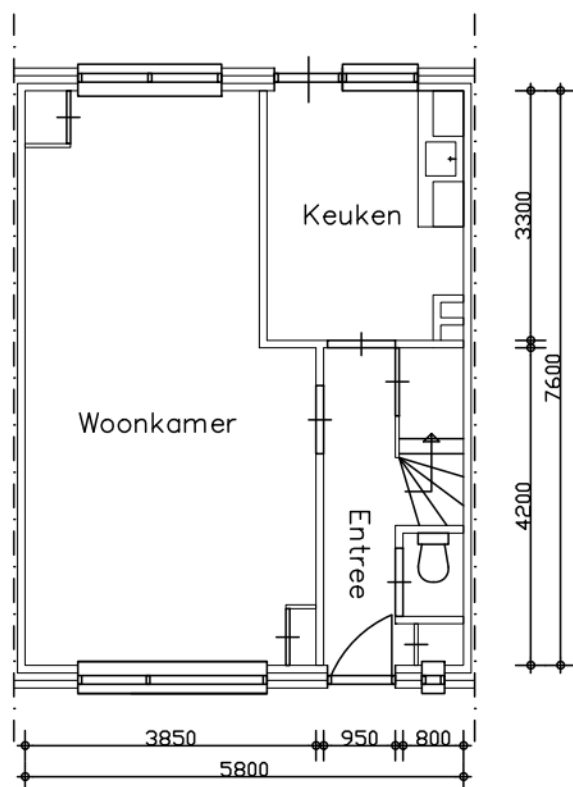
Begane grond
