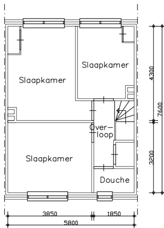
Verdieping
