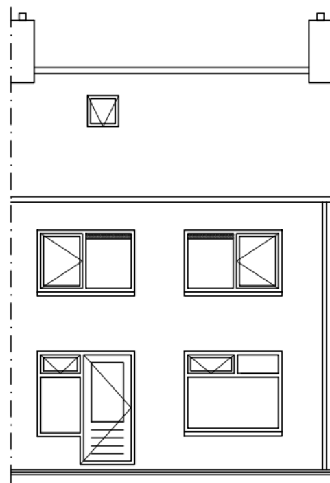
Achtergevel
