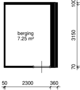
begane grond
