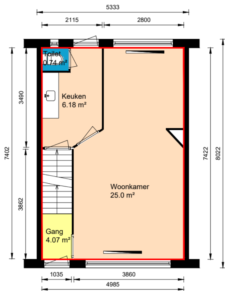
Begane grond
