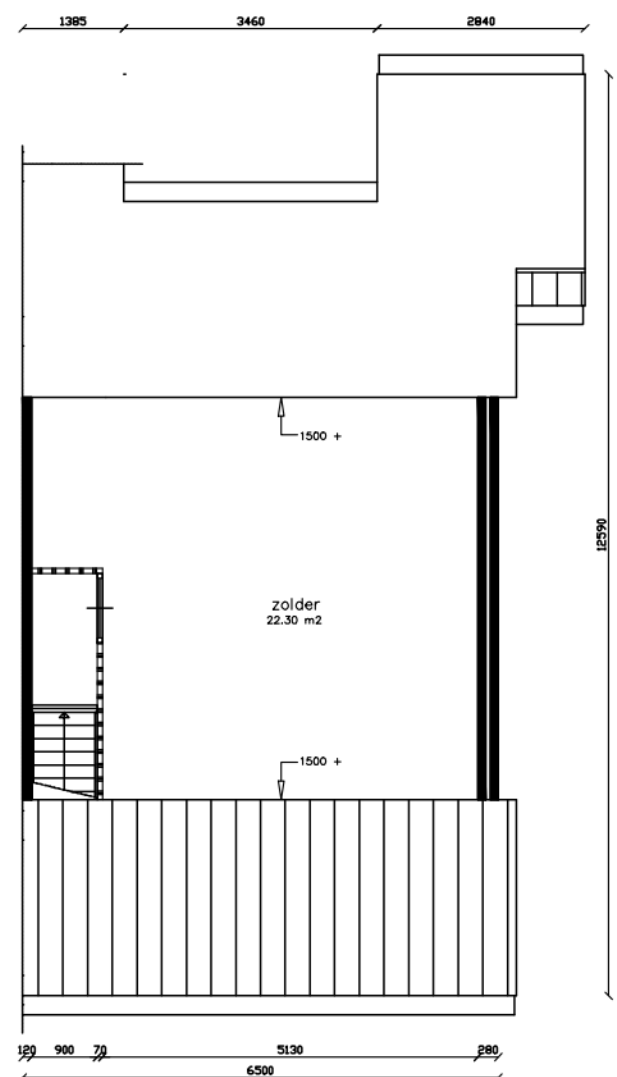
Verdieping
