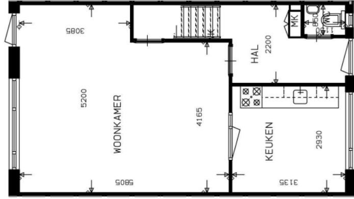
BEGANE GROND
