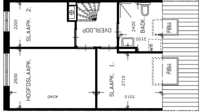
1e VERDIEPING
