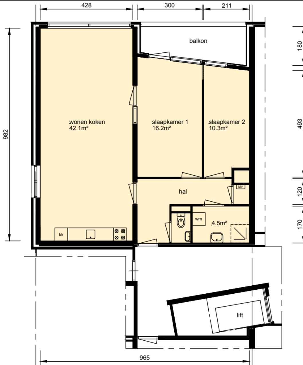
gebruiksoppervlak woonfunctie 86.68m 2 verdieping
