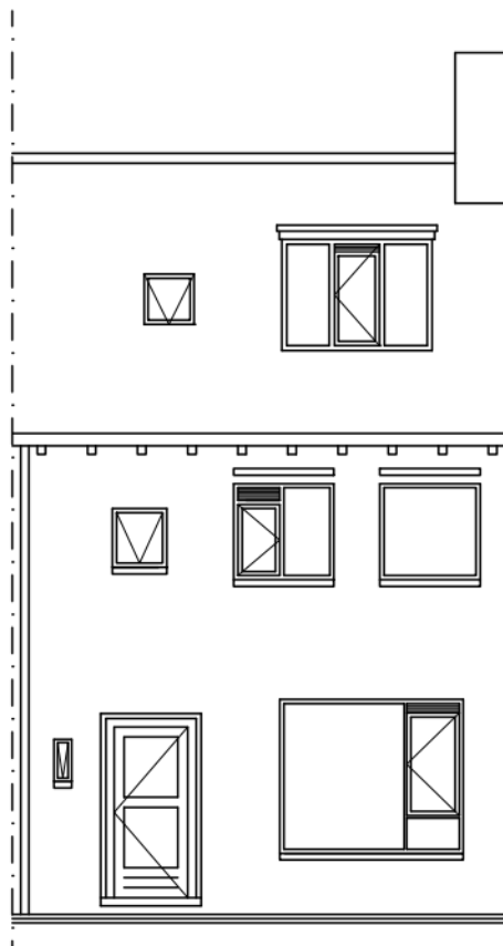
Voorgevel
