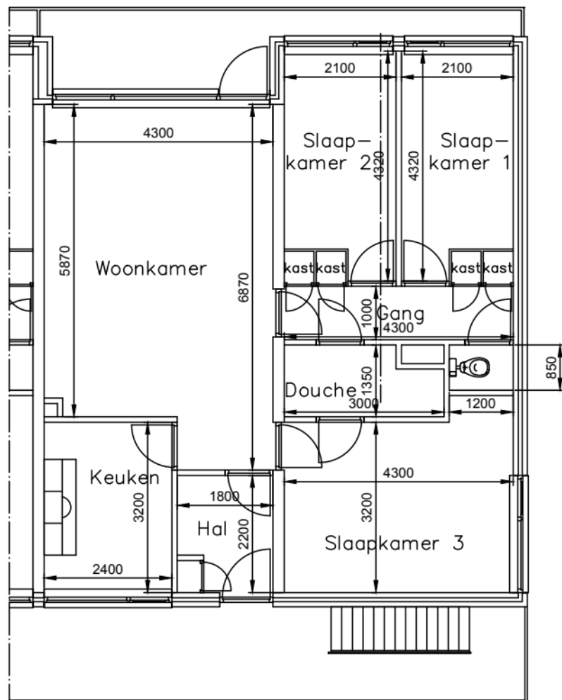
Plattegrond
