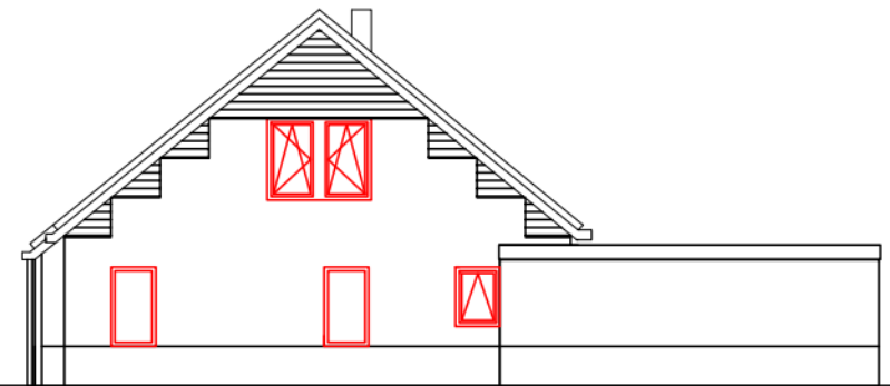
RECHTER ZIJGEVEL
