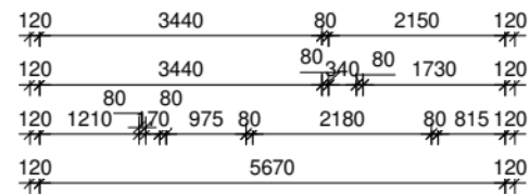
eerste verdieping
