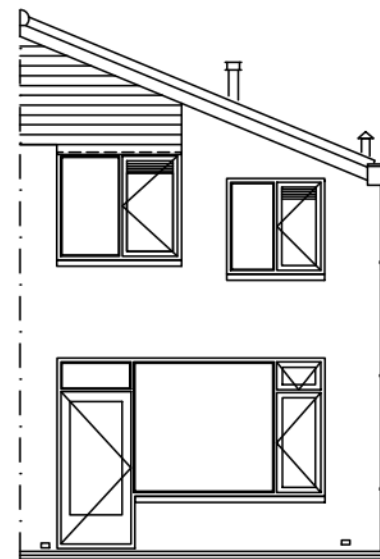
Achtergevel
