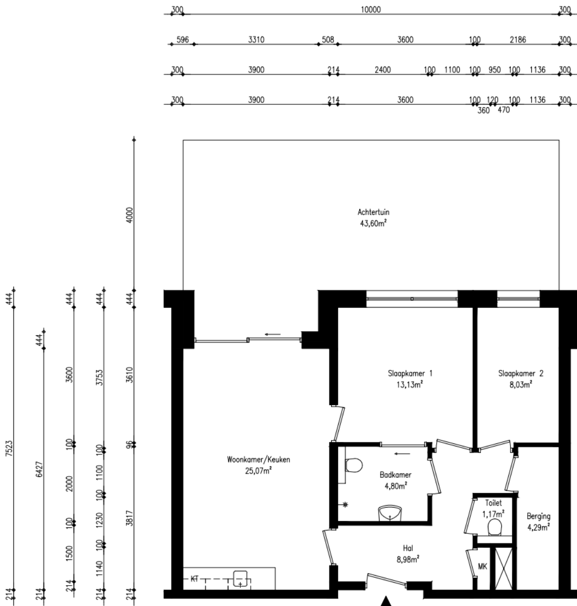
Begane grond
